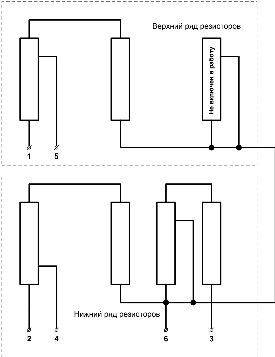
Клеммник
